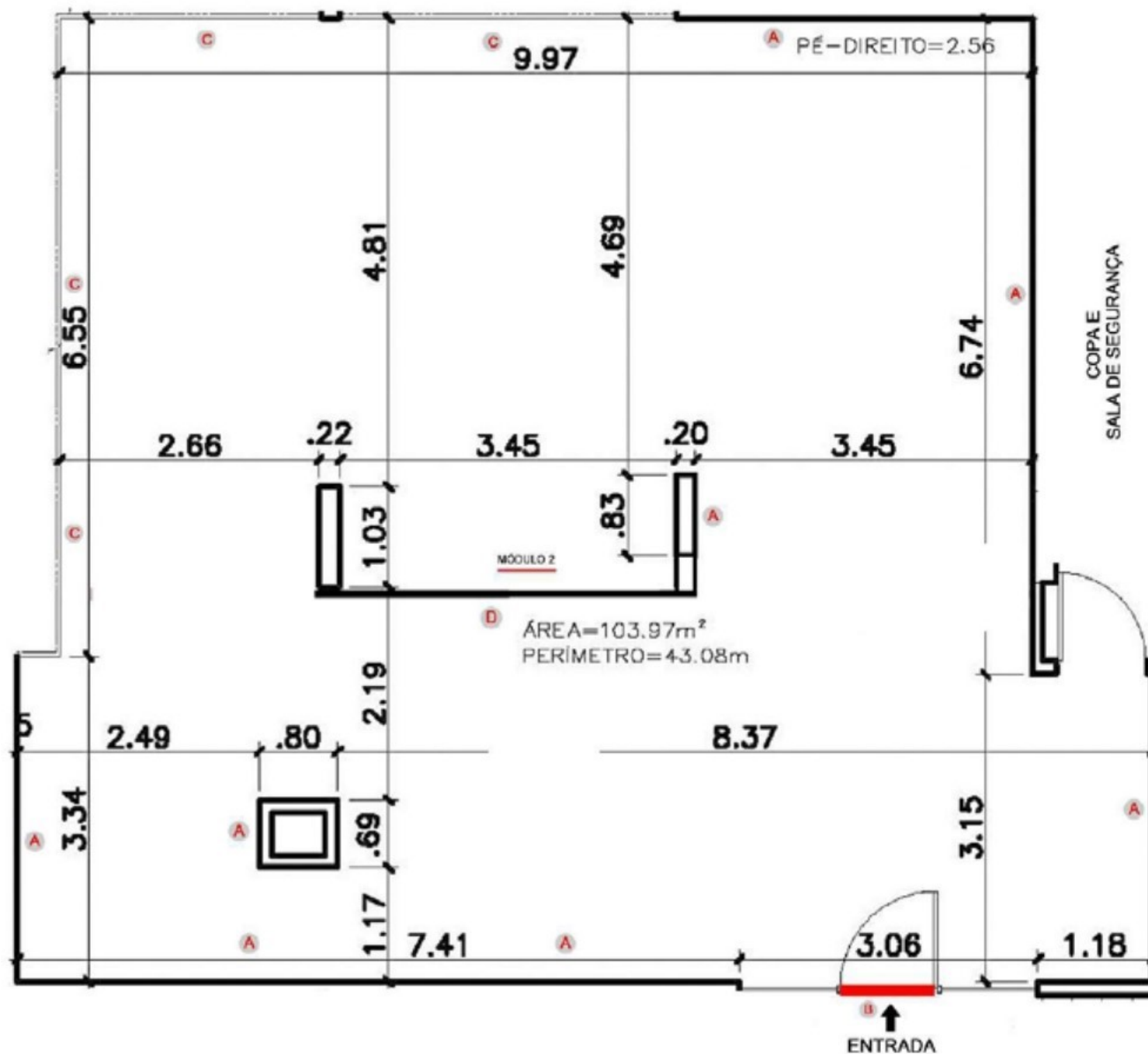
1 PLANTA BAIXA - GALERIA CAL (SUB-SOLO) ESCALA: 1:100
